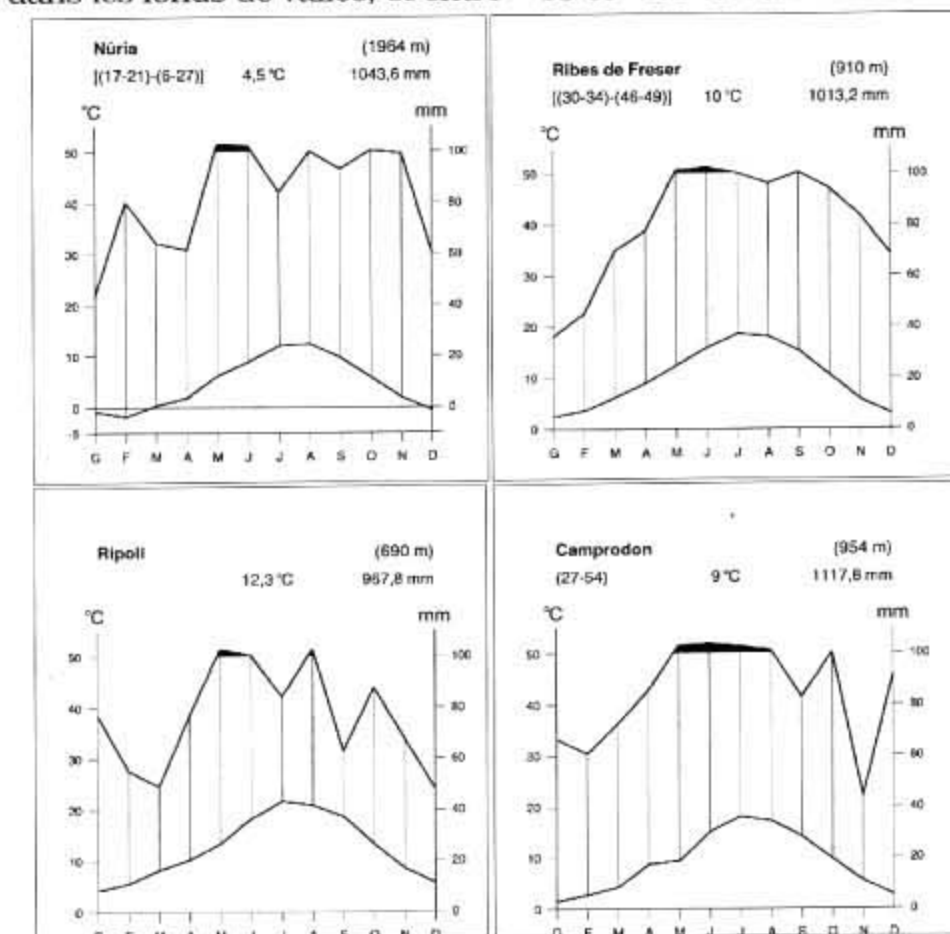
Figure 4 : Diagrammes ombrothermiques
