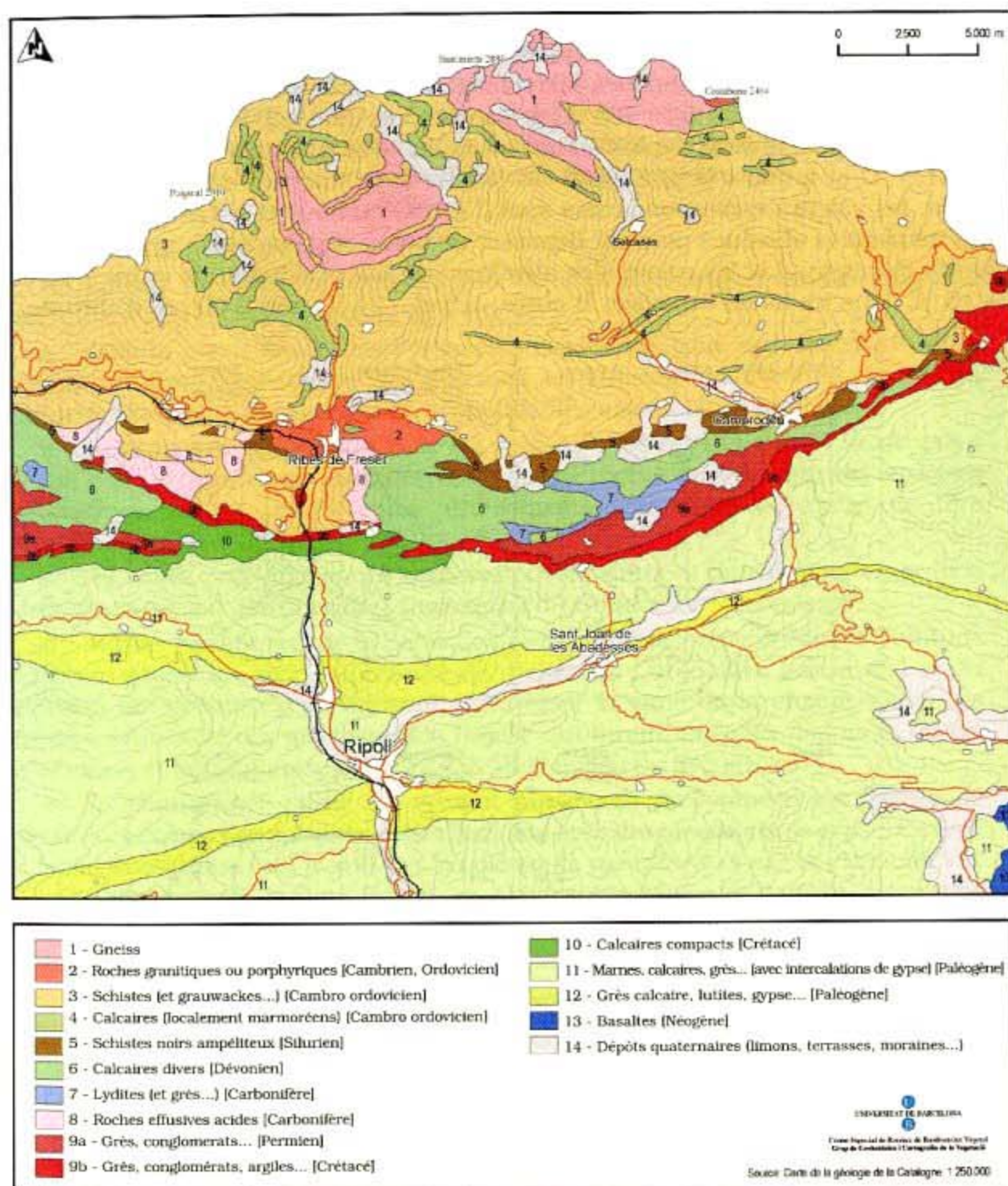
Figure 3 : Carte géologique
